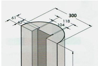
Schutzprofil Serie PUX1000 (für Stahlträger)
