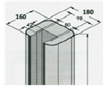
Schutzprofil Serie PUX400 (für Regalprofile / Ständerrahmen)
